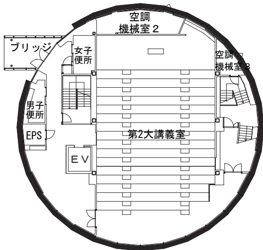
3階平面図
