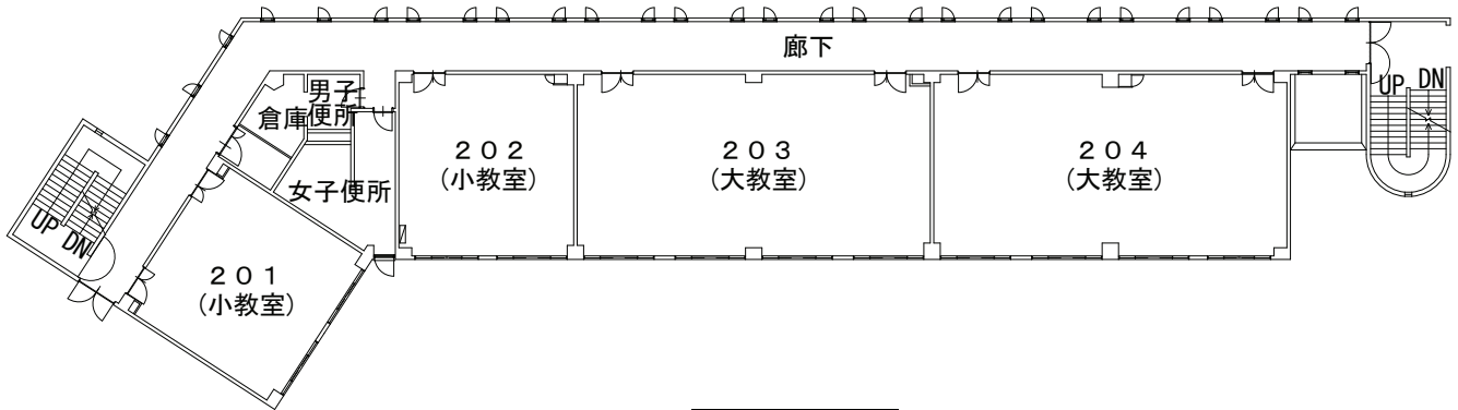
2階平面図
