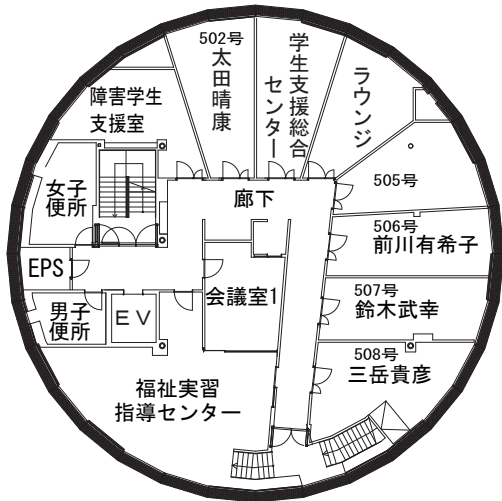
5階平面図
