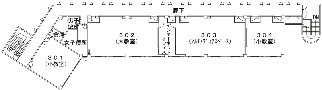
3階平面図
