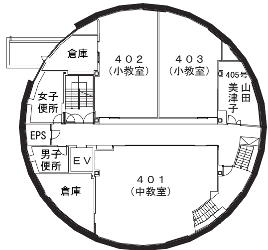
4階平面図
